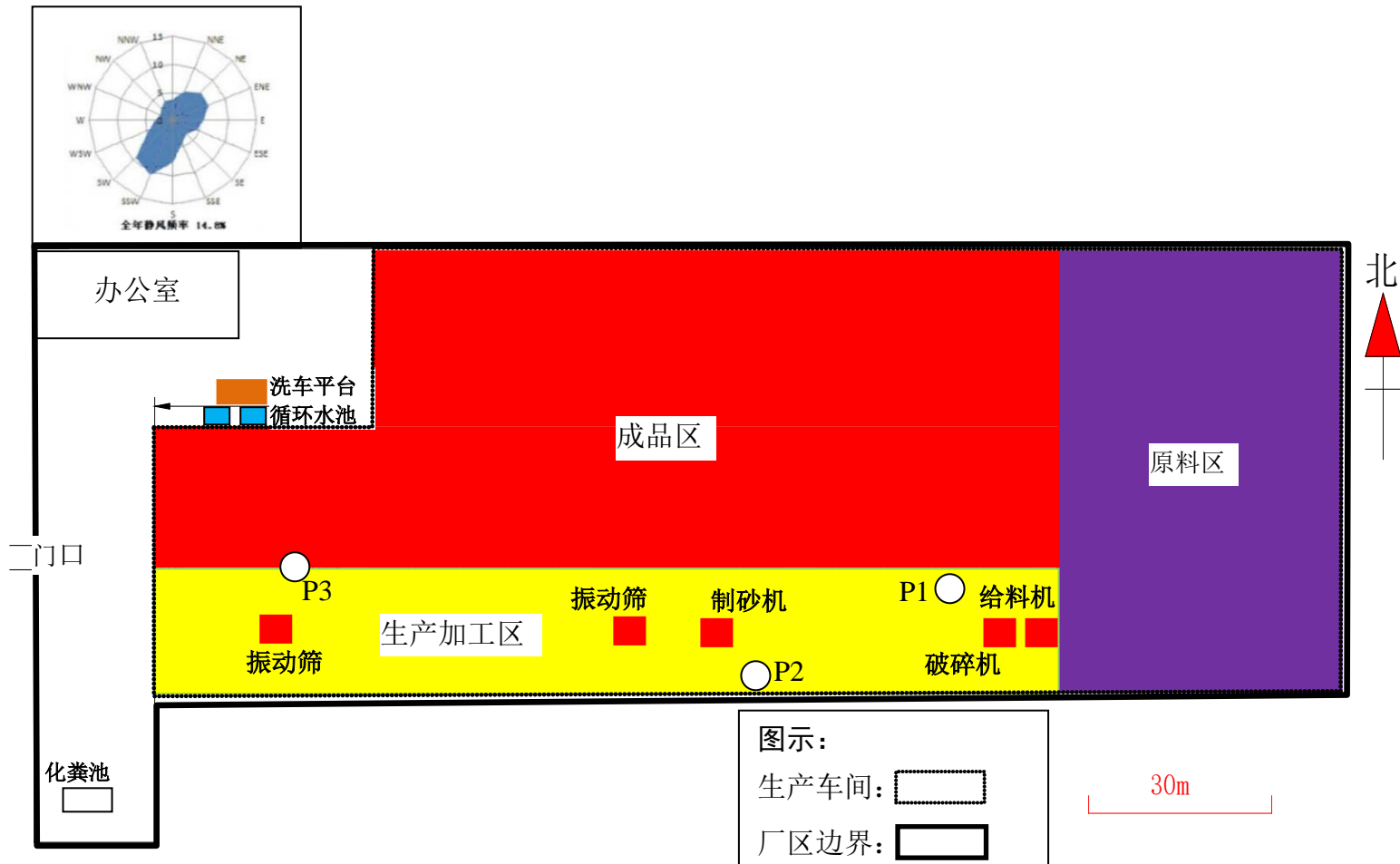
图 3.1-2 项目厂区平面布置图
