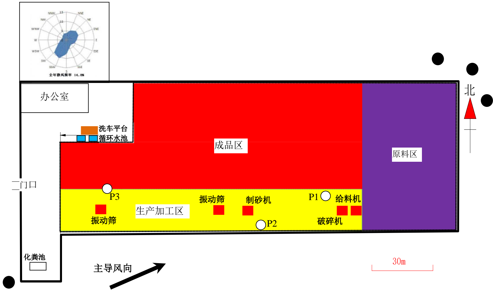
图 7.1-1 项目无组织废气监测布点图
