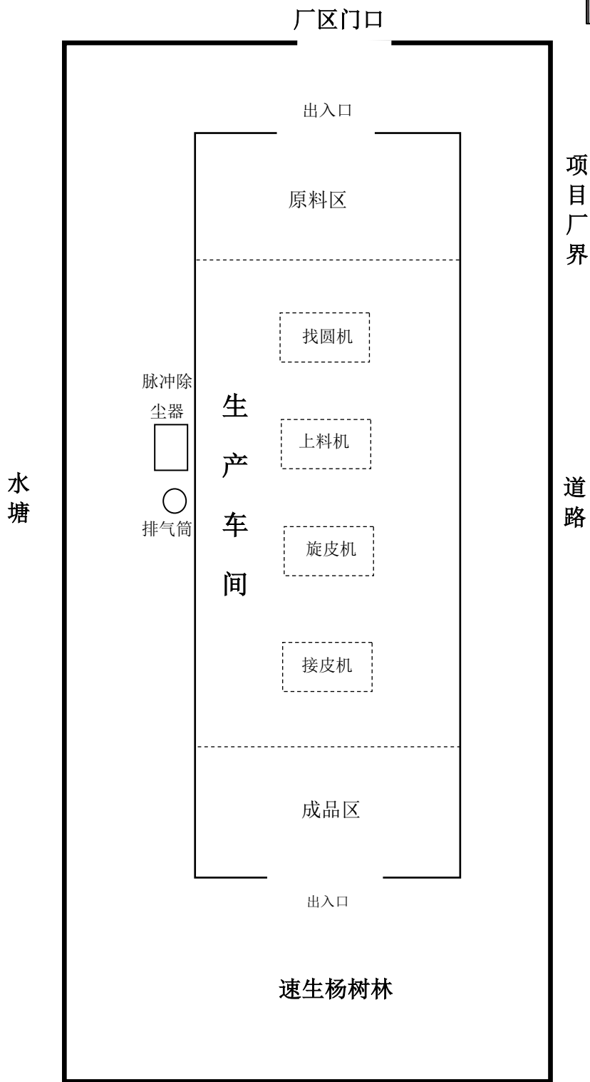
图 3.1-2 项目厂区平面布置图 (1: 200)
