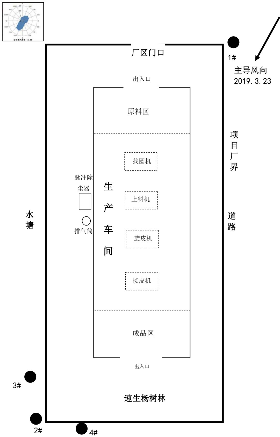
图 9.2-1 项目无组织废气监测点位示意图 (1: 200)
