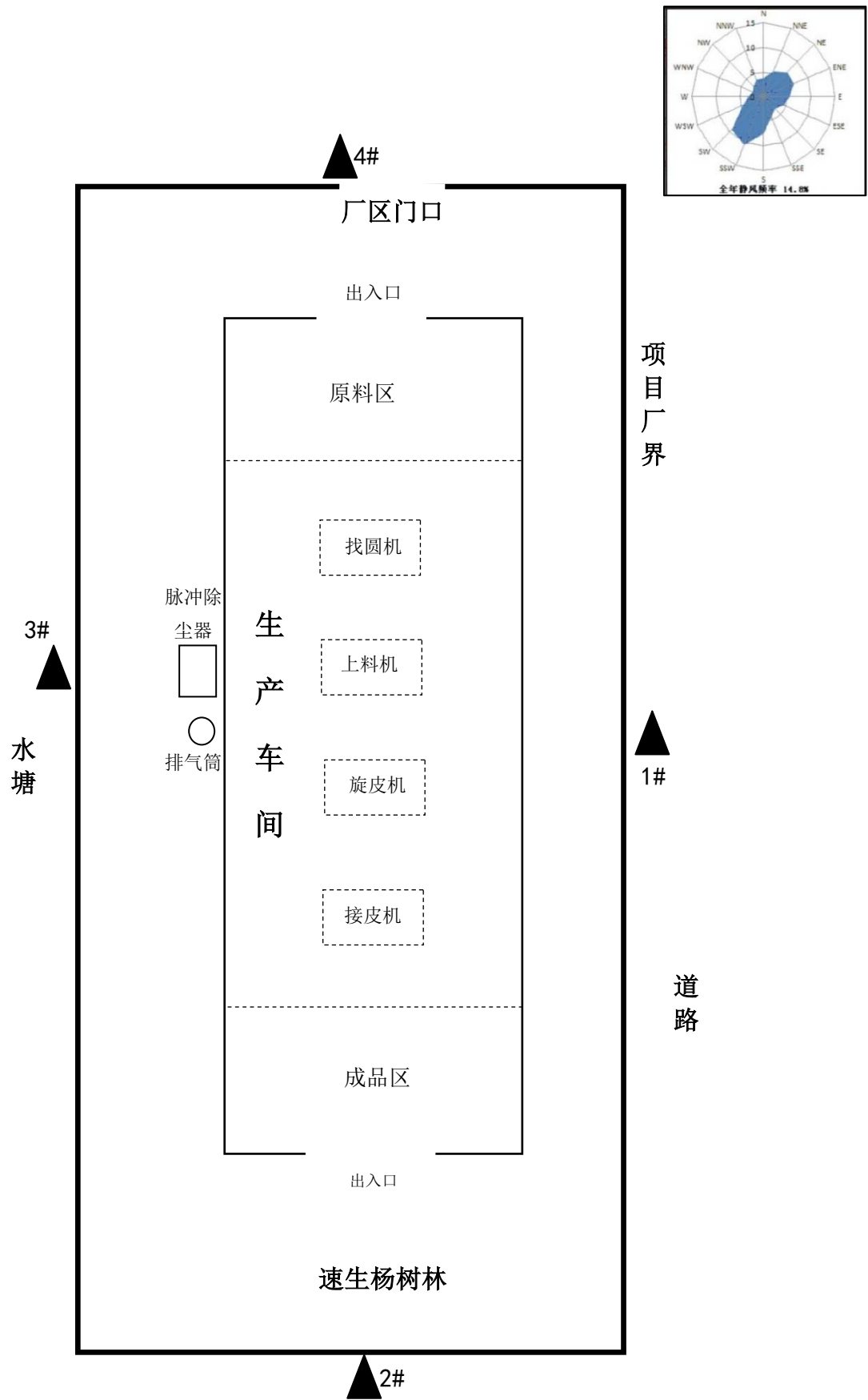
图 9.2-2 项目厂界噪声监测点位示意图 (1: 200)
