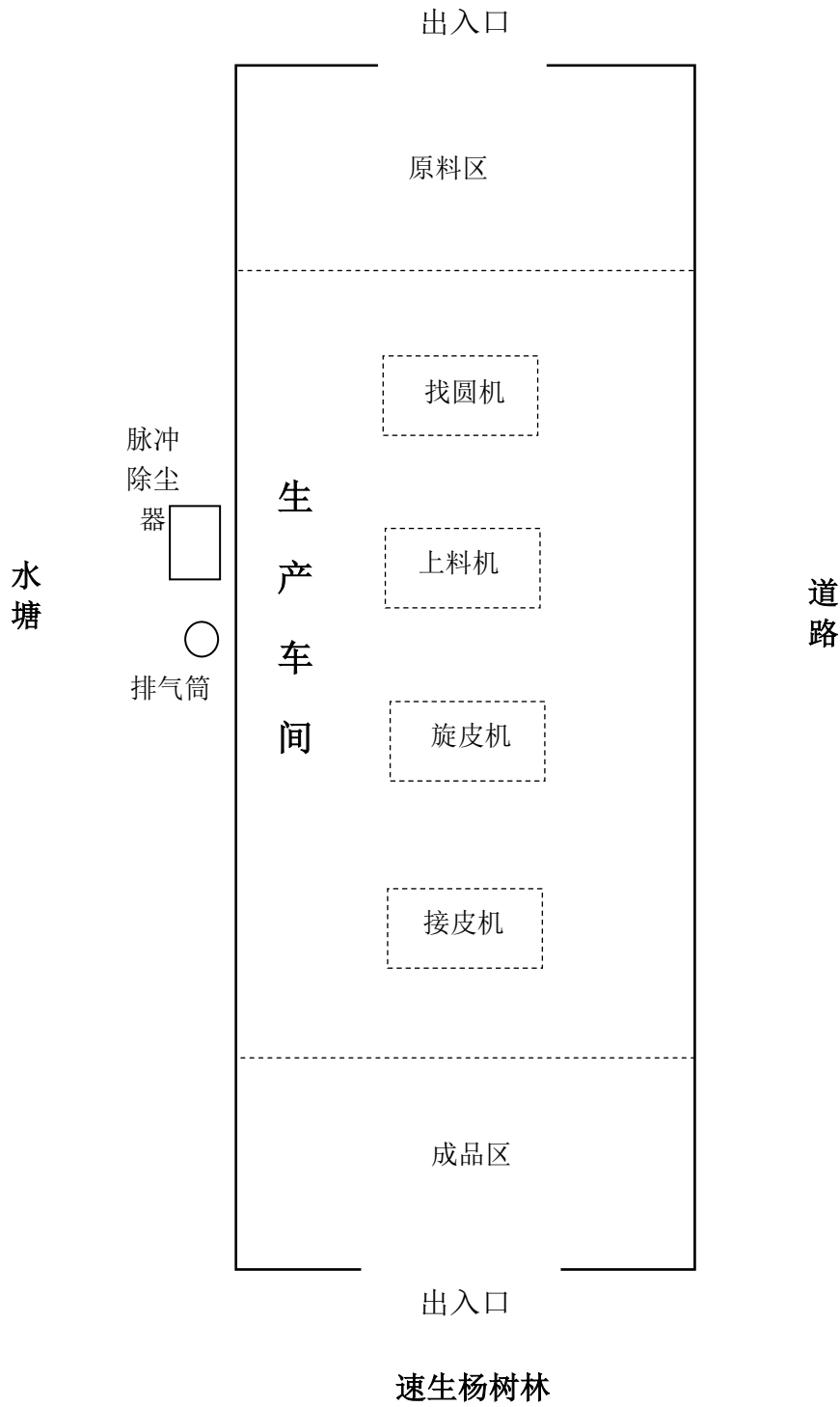
图 3.1-3 项目车间平面布置图 (1: 100)
