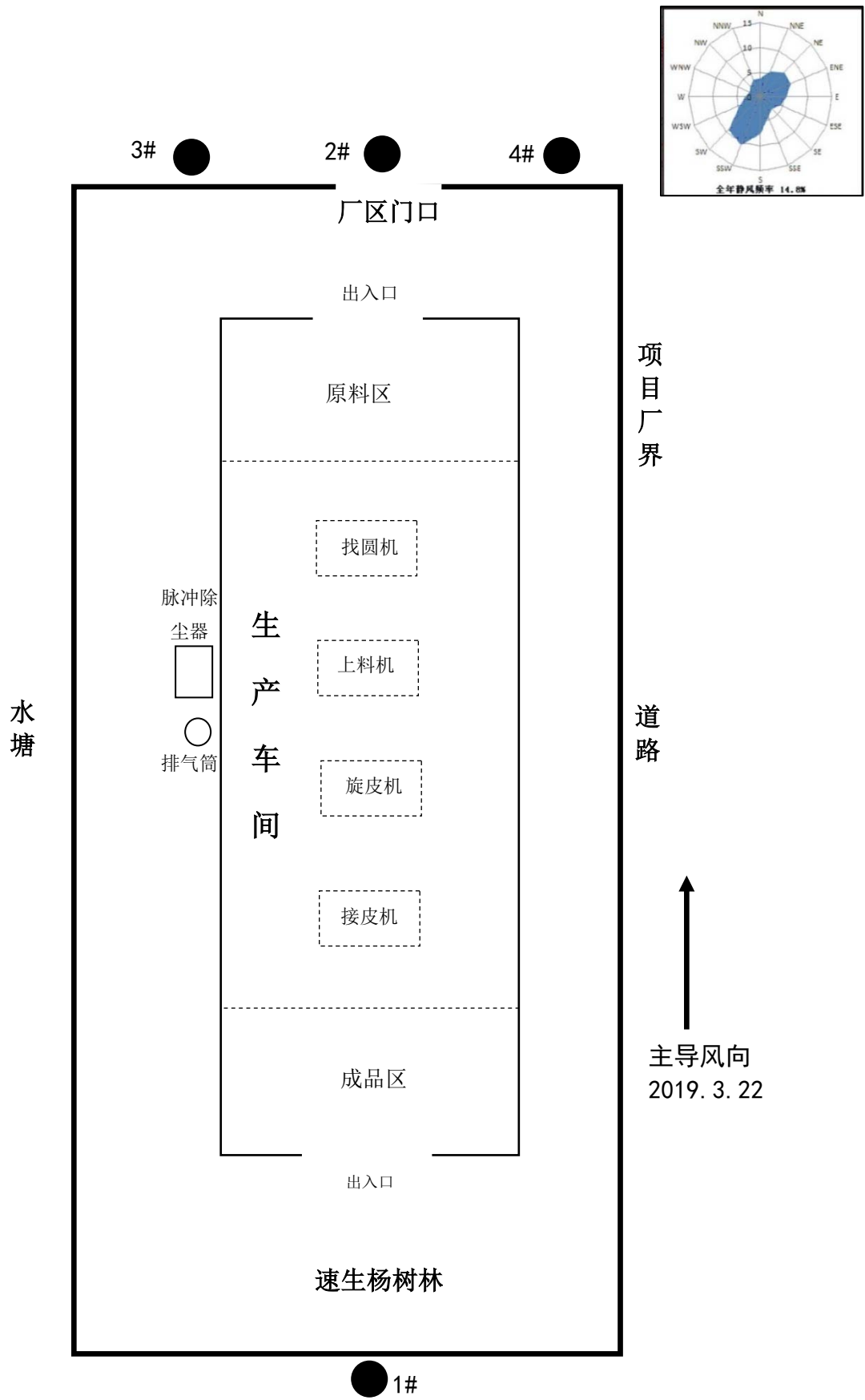
图 9.2-1 项目无组织废气监测点位示意图 (1: 200)
