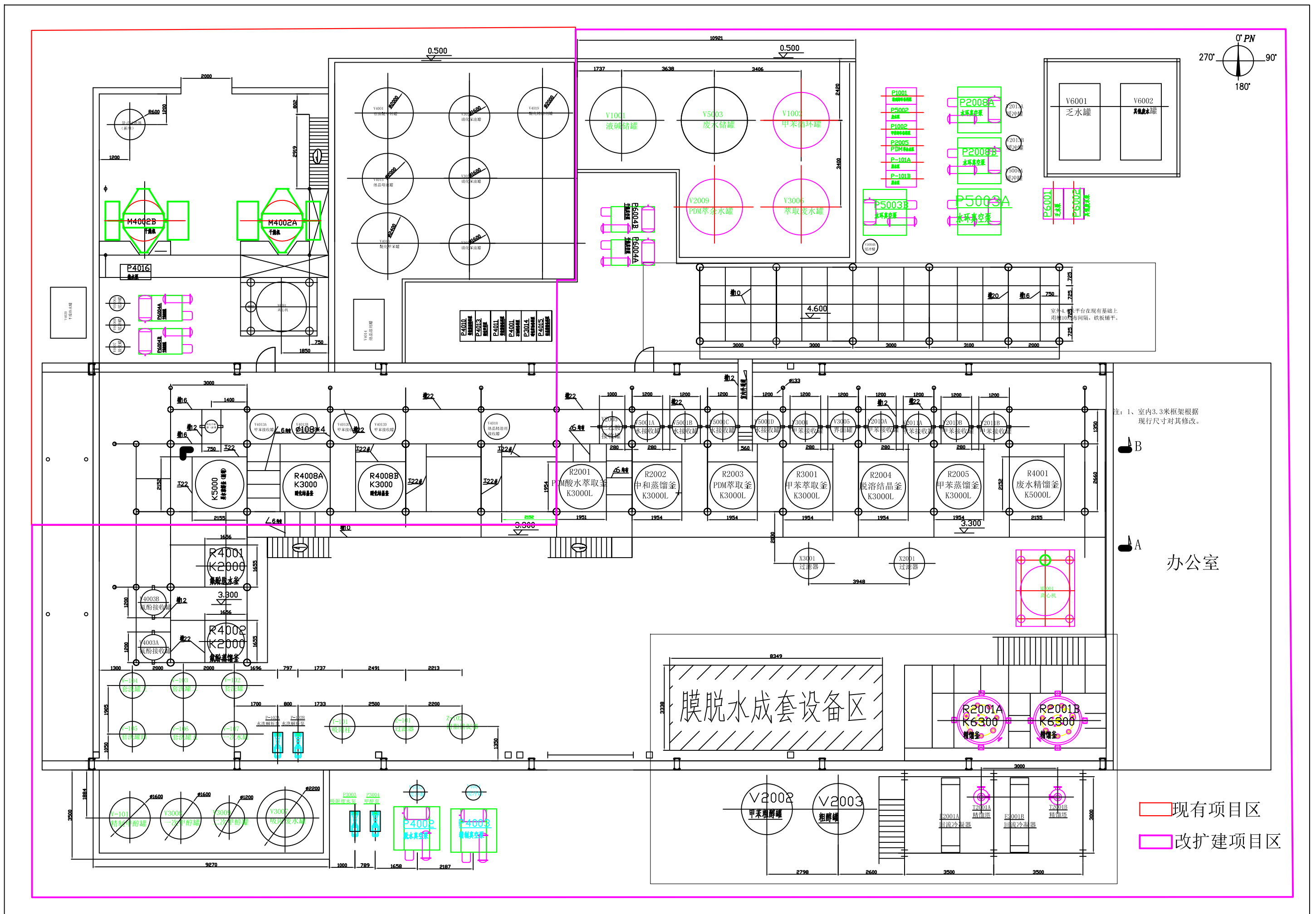
图3.1-4 项目生产车间平面布置图
