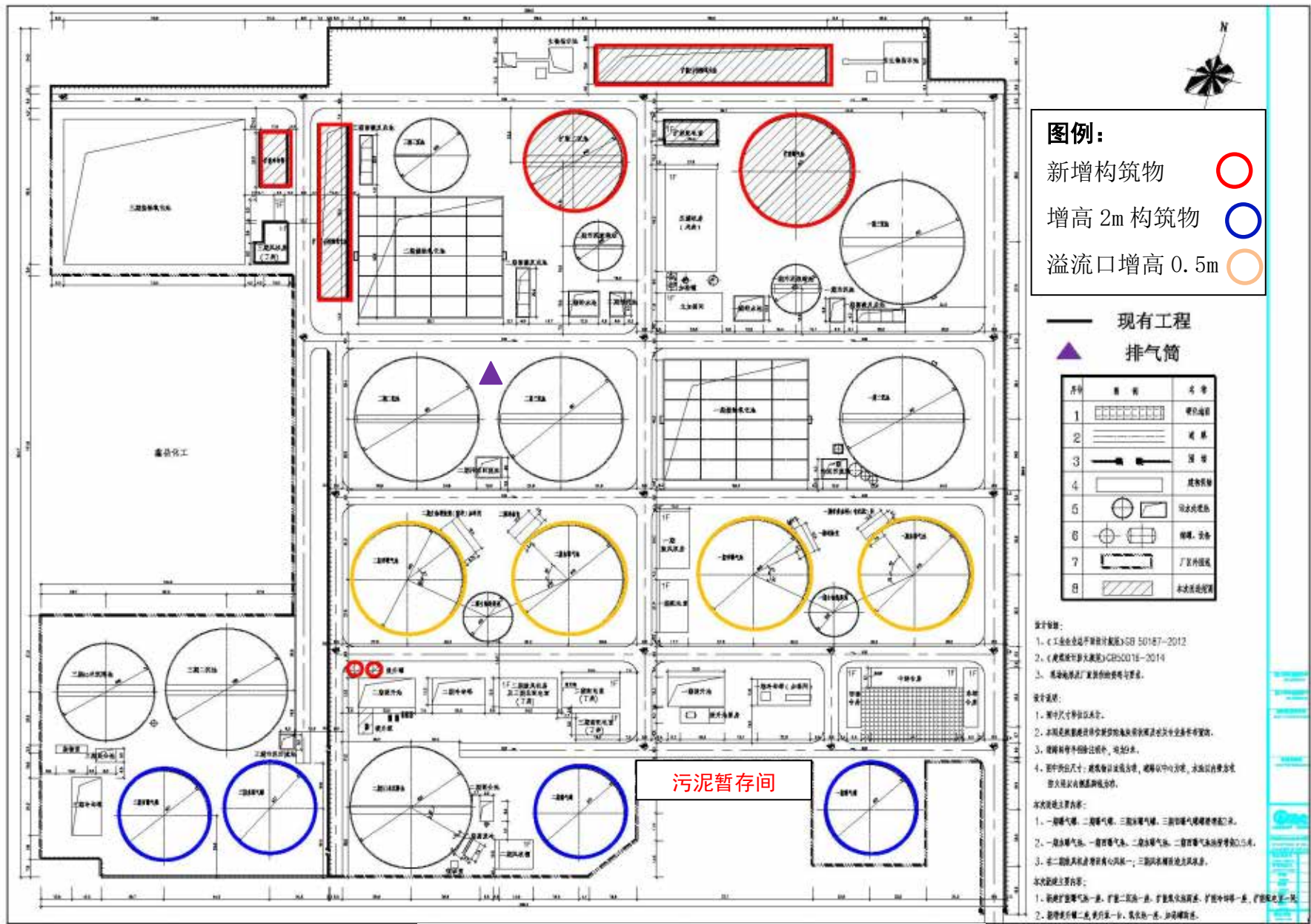
图 3.1-3 项目厂区平面布置图
