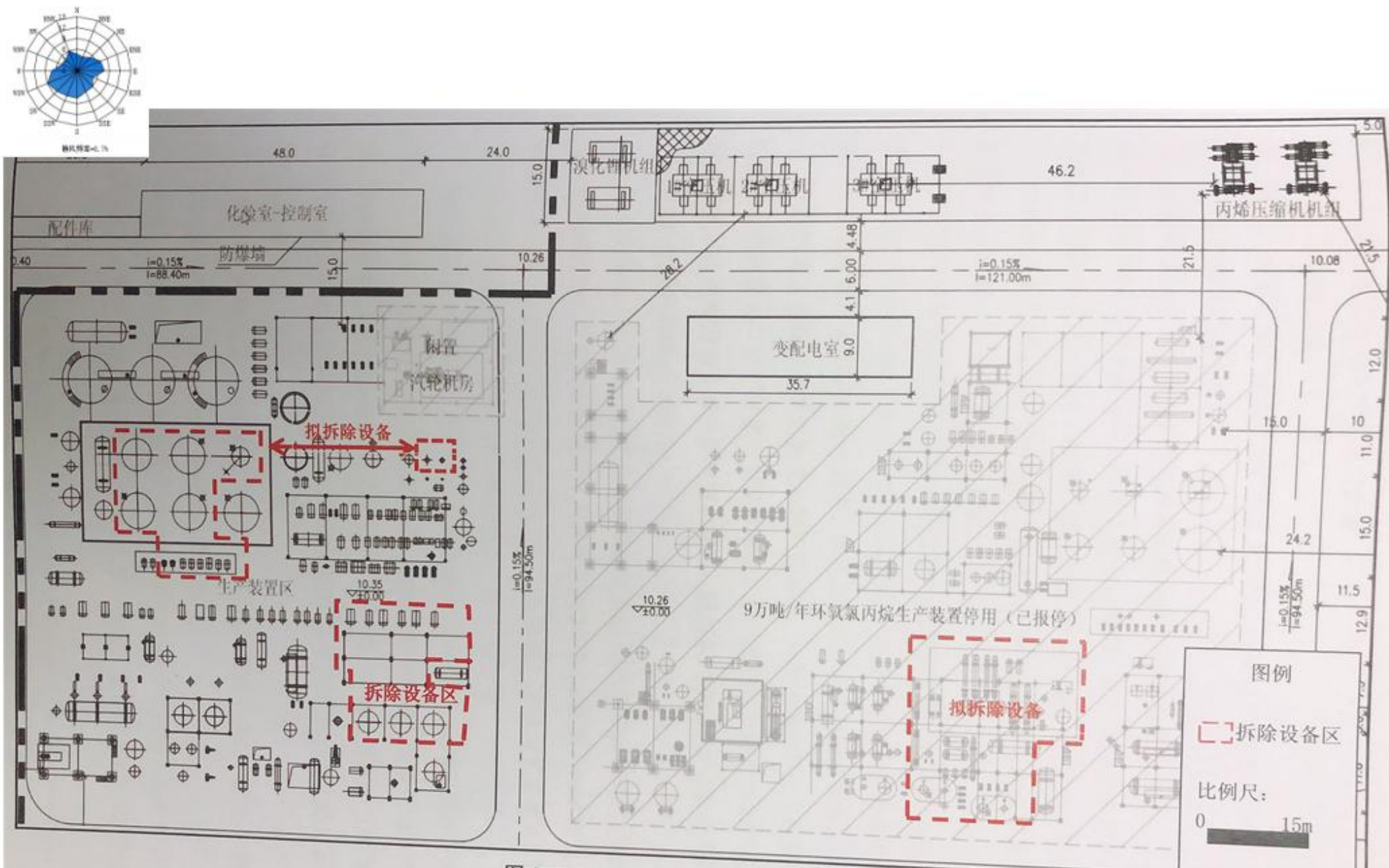
图 3.1-3 (3) 拆除设备平面布置图
