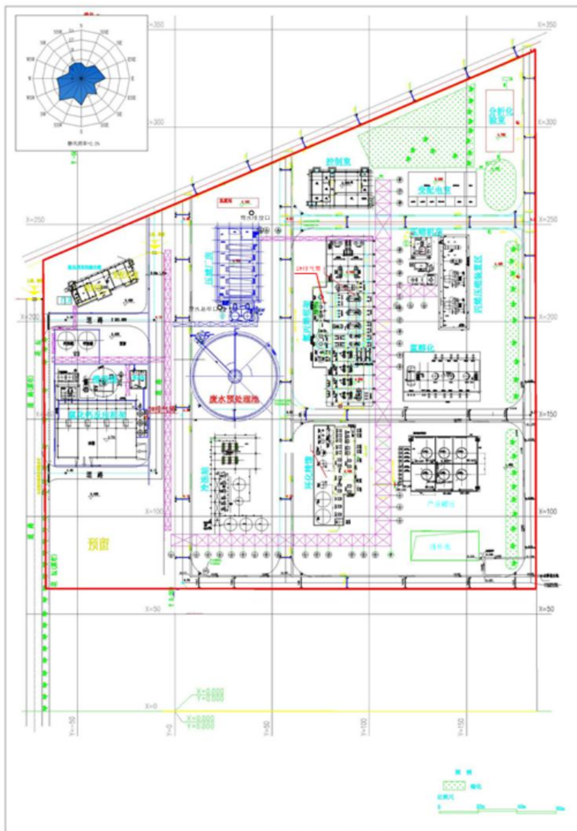
图 3.1-3 (1) 厂区总平面布置图
