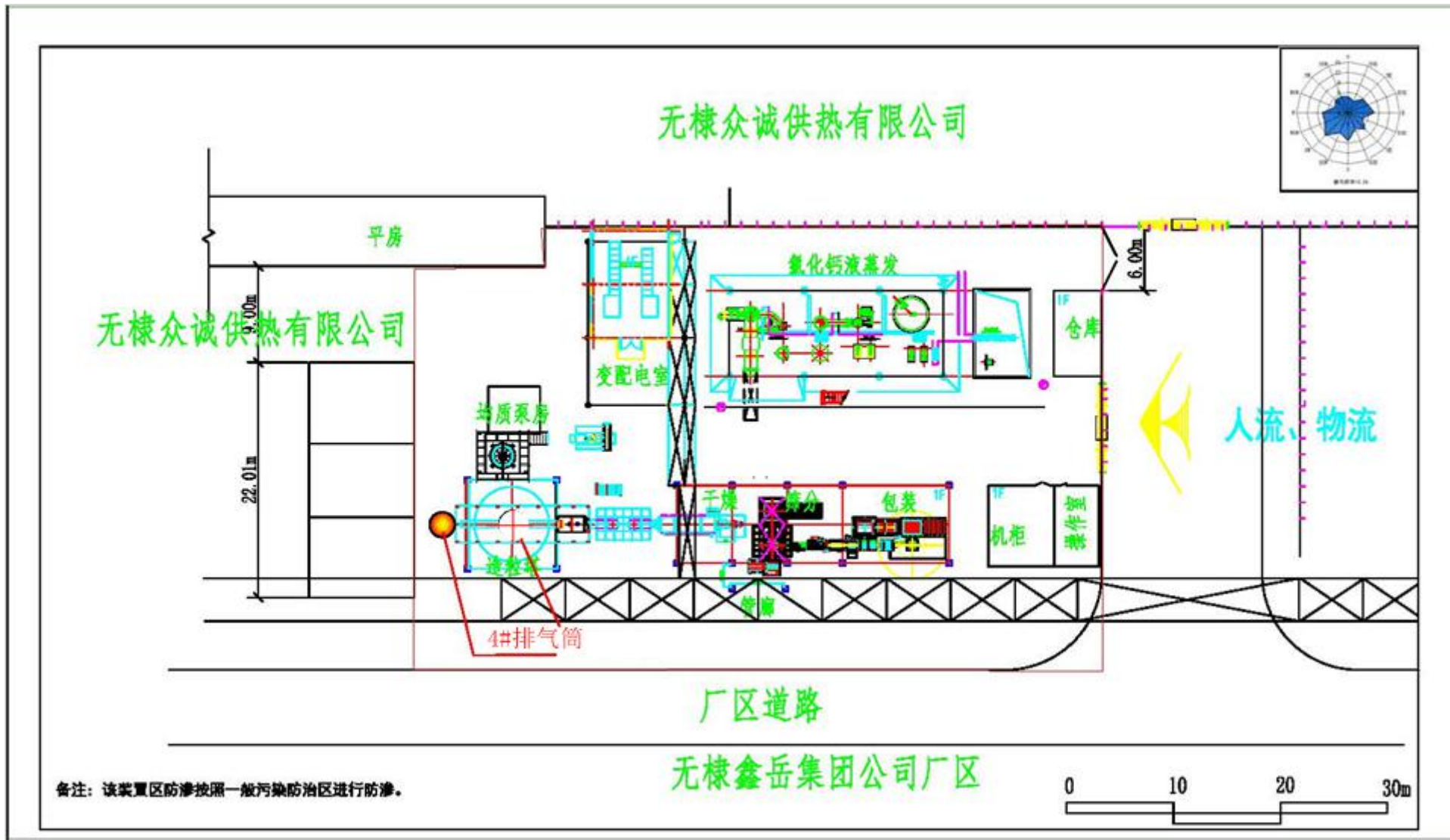
图 3.1-3 (2) 氯化钙蒸发、造粒平面布置图
