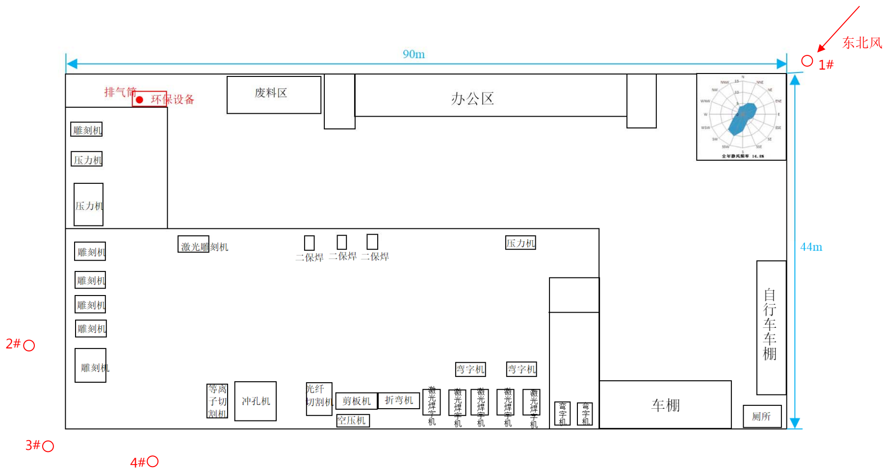
附图 7.1-1b 2018 年 7 月 11 日无组织废气监测布点图
