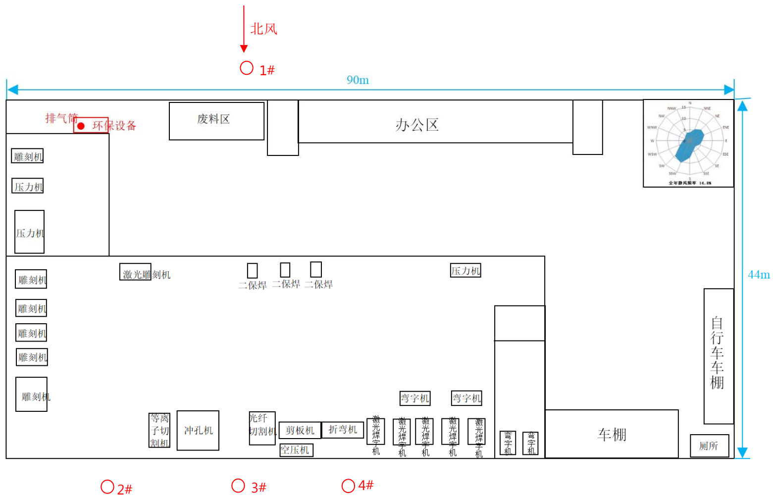
附图 7.1-1a 2018 年 7 月 10 日无组织废气监测布点图
